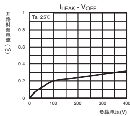
开路时漏电流—负载电压
