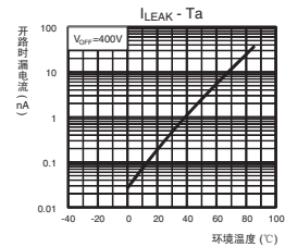
开路时漏电流—环境温度
