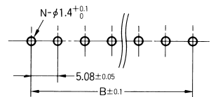
印刷基板加工尺寸 (BOTTOM VIEW)
