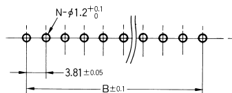
印刷基板加工尺寸 (BOTTOM VIEW)
