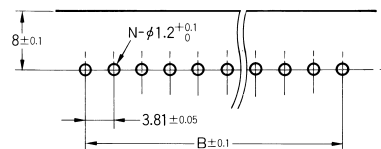
印刷基板加工尺寸 (BOTTOM VIEW)
